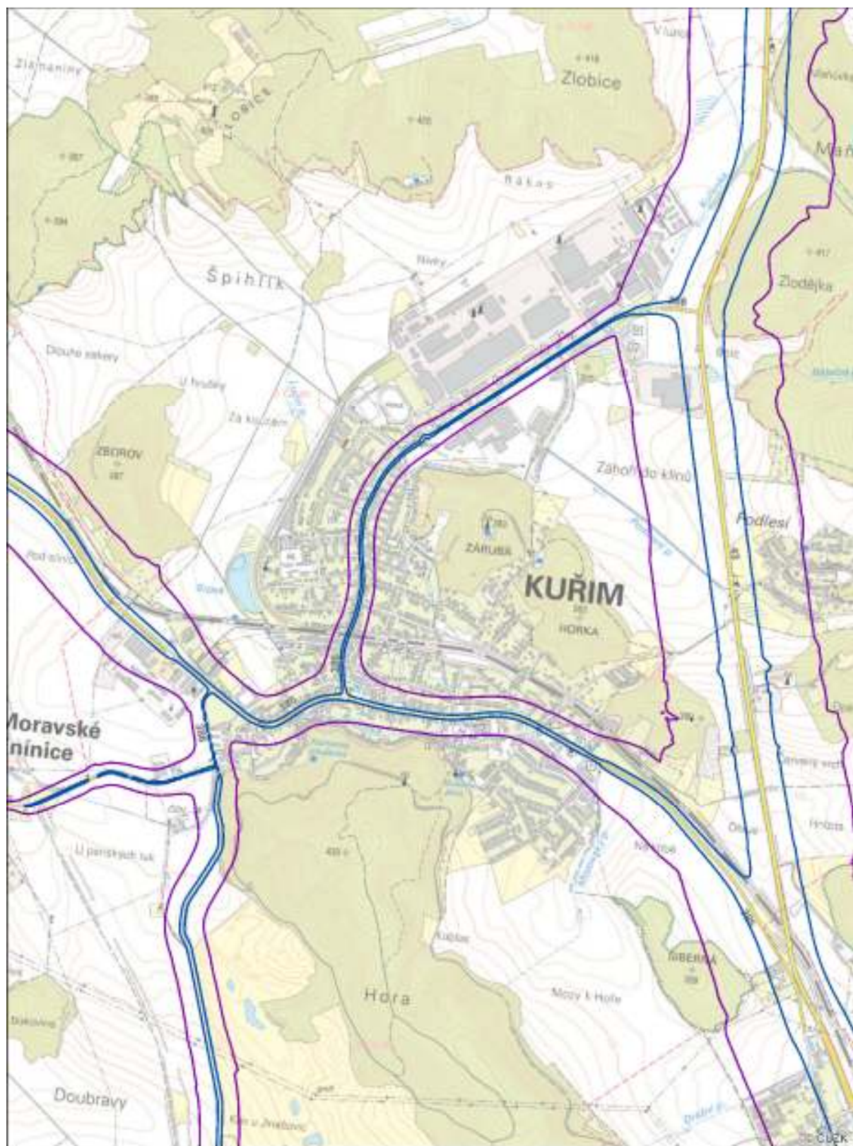
Obr. 3.28: Hluková zátěž Kuřim (noční doba) (zdroj dat: Bucek s.r.o.)
