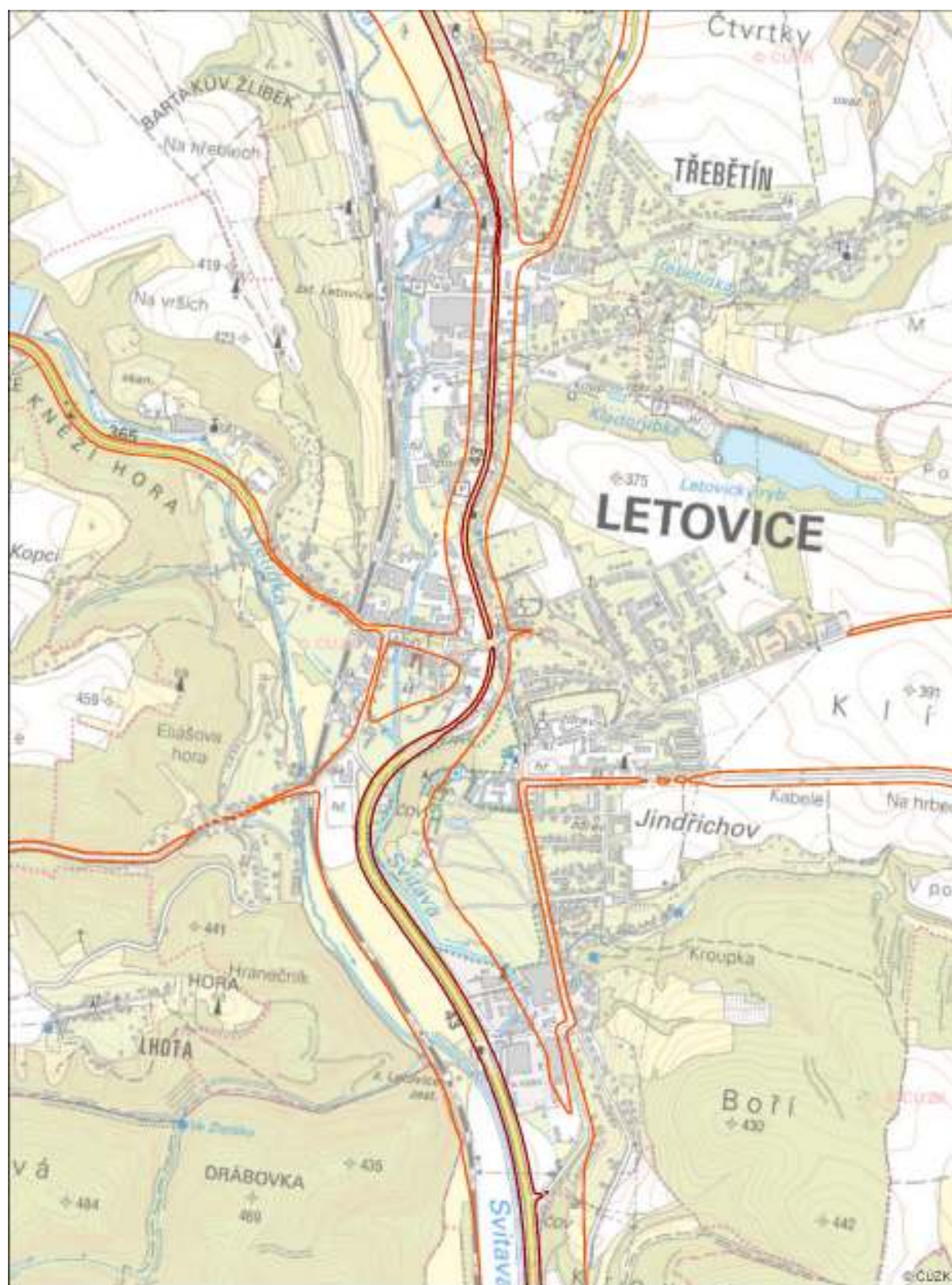
Obr. 3.29: Hluková zátěž Letovice (denní doba) (zdroj dat: Bucek s.r.o.)
