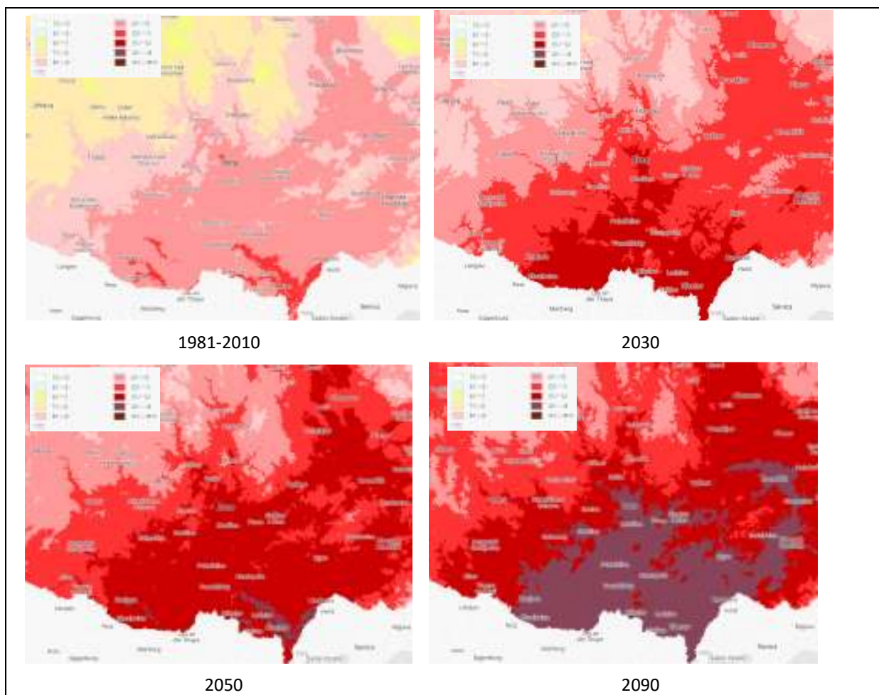
Obr. 3.54: Predikovaná průměrná roční teplota vzduchu ve třech předpovědních obdobích dle CzechAdapt (zdroj dat: CzechAdapt 2019)
