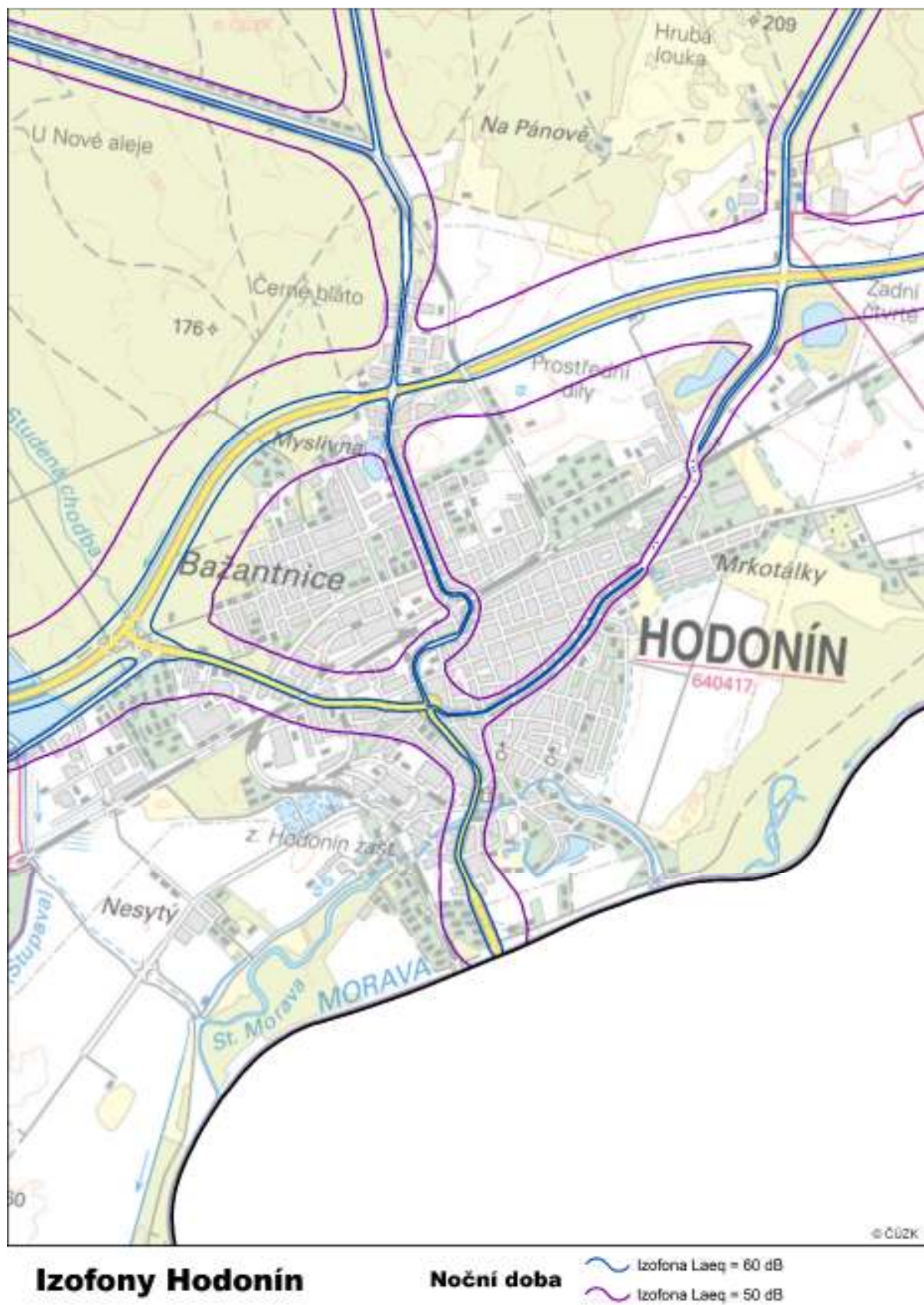
Obr. 3.32: Hluková zátěž Hodonín (noční doba) (zdroj dat: Bucek s.r.o.)
